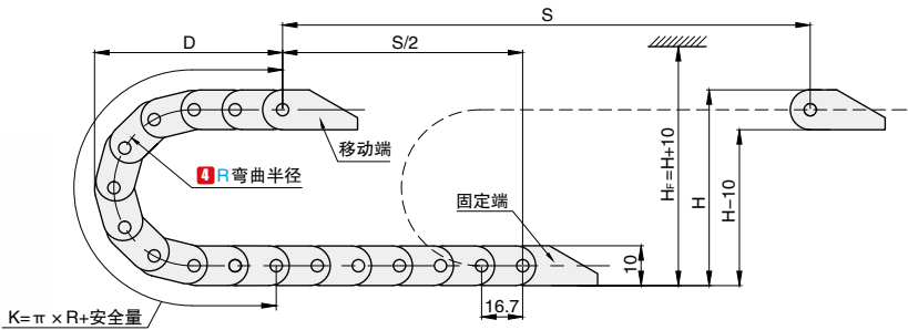
DMT07BN 不可打开型 ▲注：链长=S/2+K, S=行程距离，K=π × R+安全量
