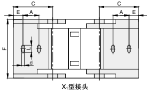
X 1 型接头
